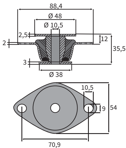
TIPO 02
