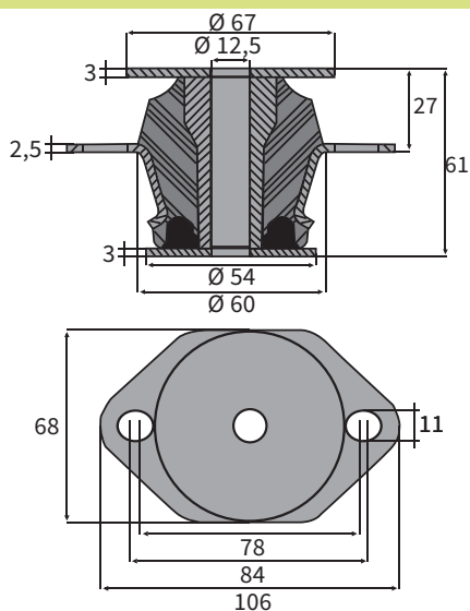
TIPO 17
