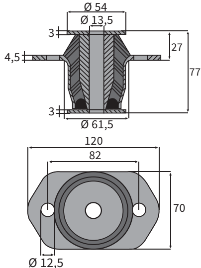
TIPO 21
