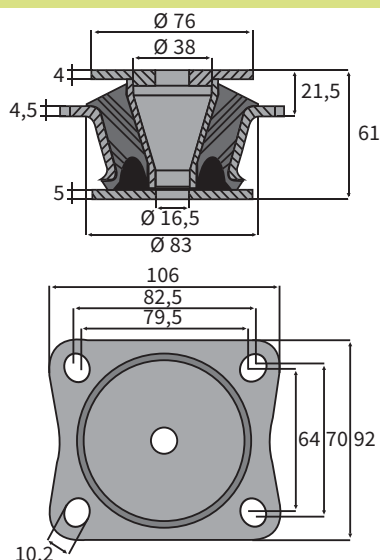
TIPO 21
