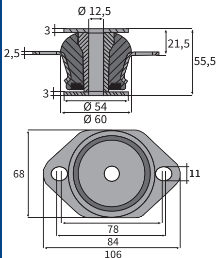
TIPO 17
