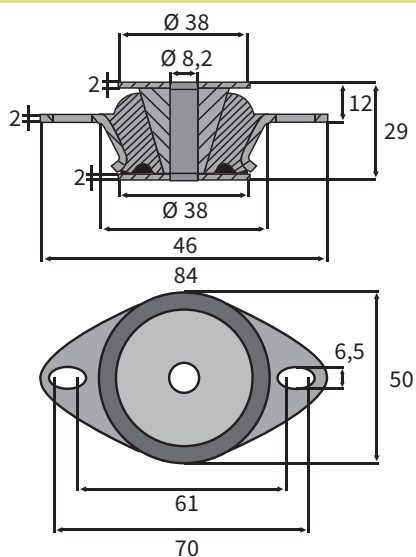
TIPO 13
