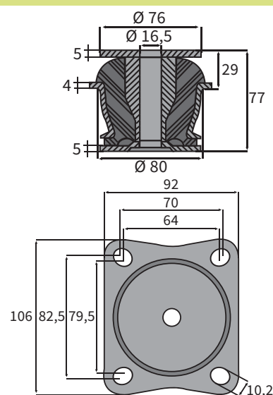
TIPO 31
