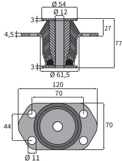
TIPO 31
